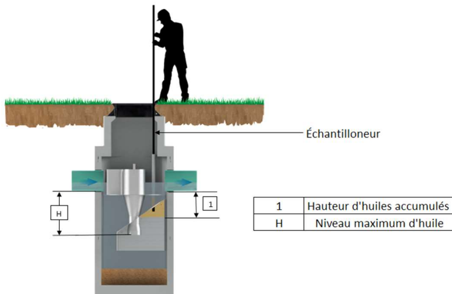
Figure 2 : Méthode d'inspection du niveau d'huile
