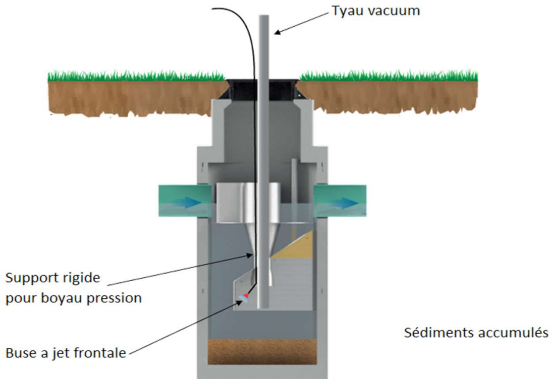
Figure 5 : Nettoyage des sédiments
