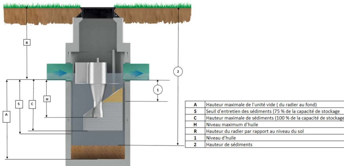
Figure 1 : Paramètres de référence pour l'entretien des SDD3
